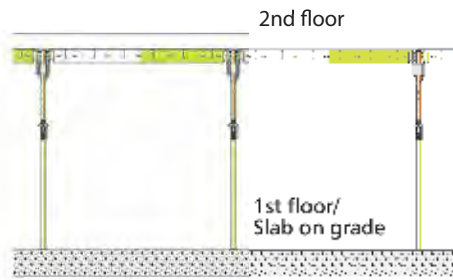
Step 2 Shoring complete, pour second floor.
